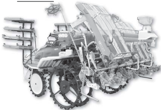
田植機
